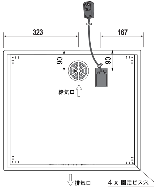
底面図
