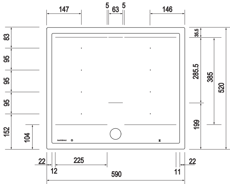
上面図
