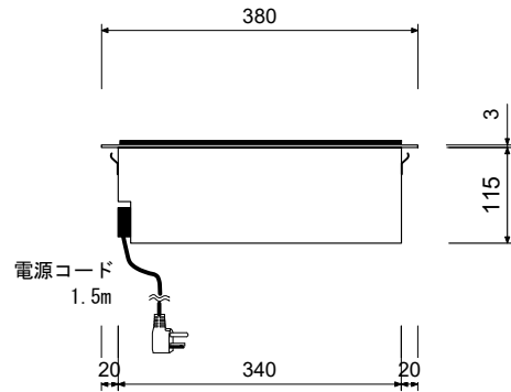
正面図
