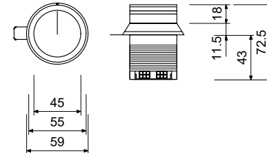
コントロールノブ
